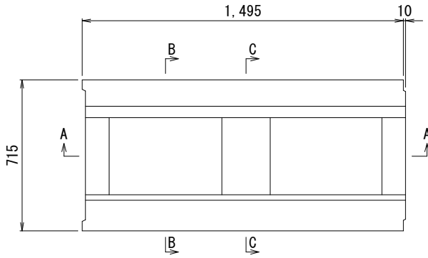
平面図
