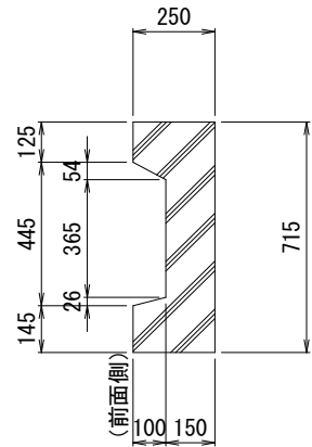
C-C断面図
