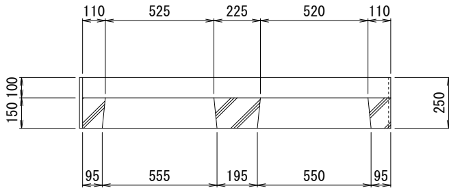
A-A断面図
