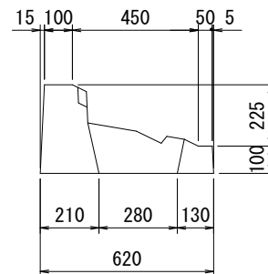
B-B断面図
