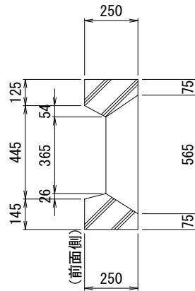
B-B断面図
