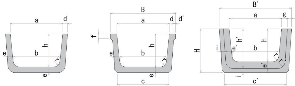
スピゴット部 断面図
