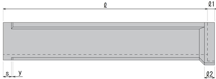
スピゴット部 断面図
