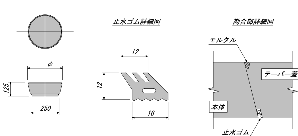
【テーパー蓋】
