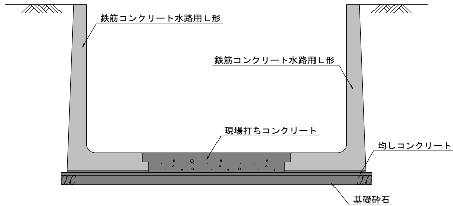
L形水路施工断面図
