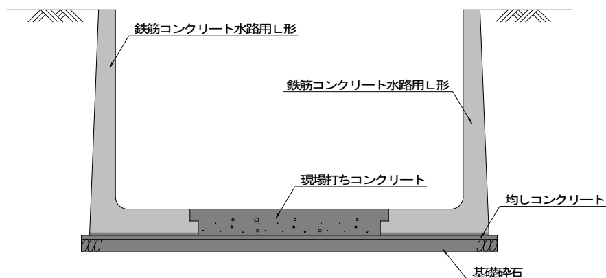
L形水路施工断面図
