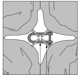
連結筋 連結金具(シャクル)
