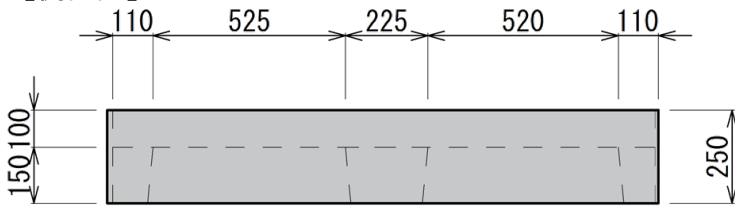
【側面図】
