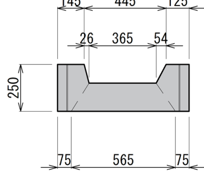
【正面図】
